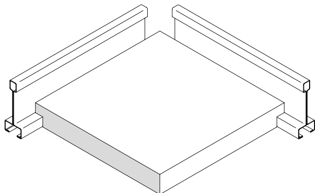
Bordo scanalato 8 mm per profilo scanalato / 8-mm grooved edge for grooved profile / Gerillte Kante 8 mm für Rillenprofil / Bord rainuré 8 mm pour profilé rainuré / Borde acanalado de 8 mm para perfil acanalado
