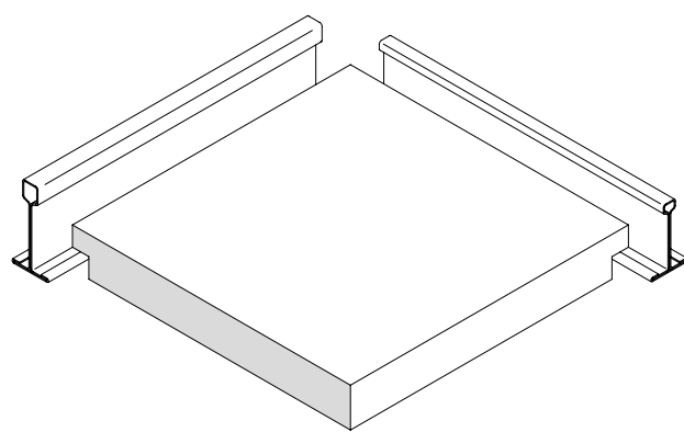
Bordo scanalato 8 mm per profilo T15 / 8-mm grooved edge for profile T15 / Gerillte Kante 8 mm für Profil T15 / Bord rainuré 8 mm pour profilé T15 / Borde acanalado de 8 mm para perfil T15
