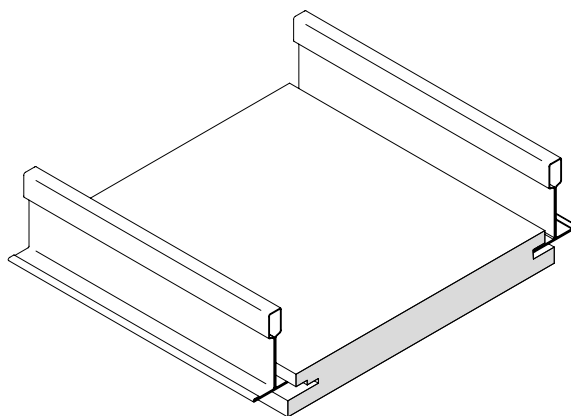
Bordo a semi-scomparsa per profilo T24 / Semi-concealed edge for profile T24 / Halb-verdeckte Kante für Profil T24 / Bord à demi-caché pour profilé T24 / Borde semiescamoteable para perfil T24
