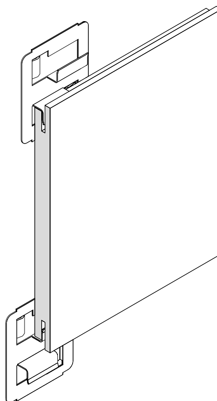
Bordo per montaggio a parete con clip di aggancio / Edge for wall-mounting with clip attachment / Kante für Wandmontage mit Clip zum Einhängen / Bord pour montage au mur avec clip de fixation / Borde para montaje en pared con clip de enganche
